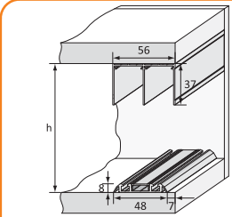
Bėgelių montavimas
