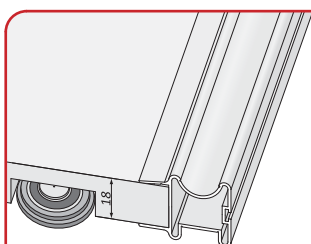
Plokštės tvirtinimas prie šoninio profilio #18mm
