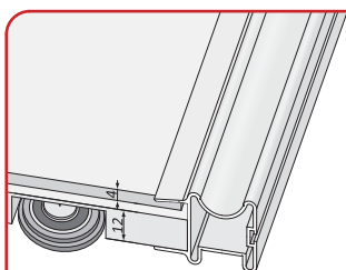
Stiklo prie šoninio profilio tvirtinimas #16mm
