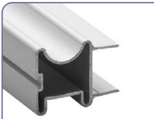
Šoninis profilis NEPTUN
