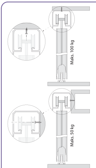
Bėgelio tvirtinimas
