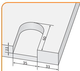
Vežimėlio lizdo frezavimas
